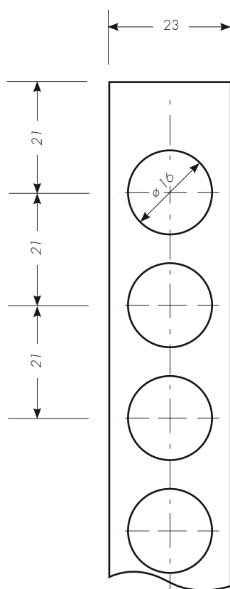
Detail „A“
