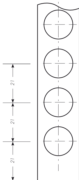
Detail „B“
